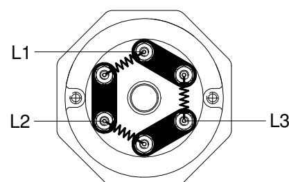
D-koppling
