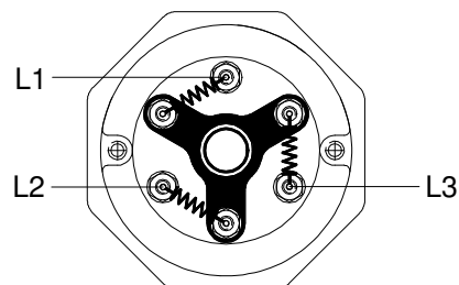
D-koppling
